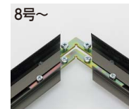
1角に2ヶ所ネジ止め
